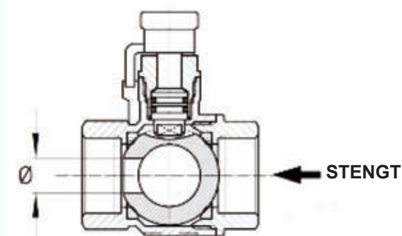
Kule med ekspansjonshull. Pilen viser ekspansjonsretning, ved stengt ventil.
